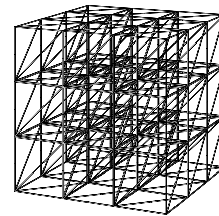
stabwerk
